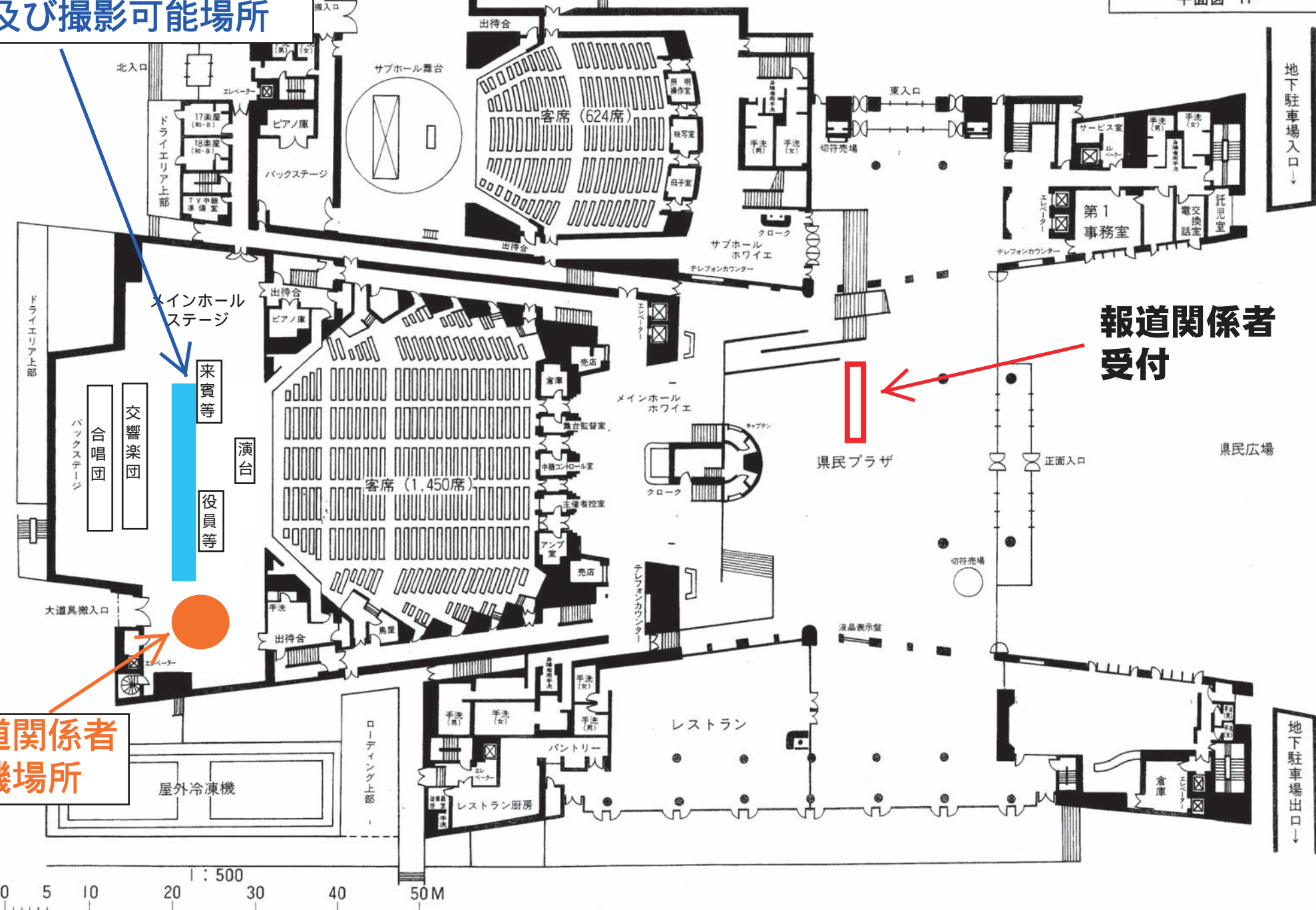
平面図 1F
